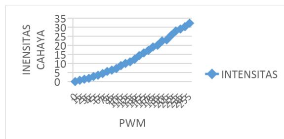
Gambar 9. Besar Intensitas Cahaya Berdasarkan Nilai PWM
