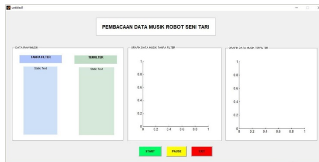
Gambar 4. Desain GUI
