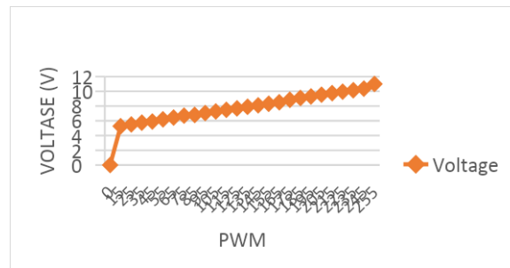
Gambar 8. Besar Voltase berdasarkan PWM
