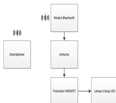
Gambar 1. Diagram Prinsip kerja sistem kontrol
