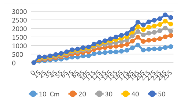
Gambar 10. Perbandingan pengukuran intensitas pada jarak tertentu
